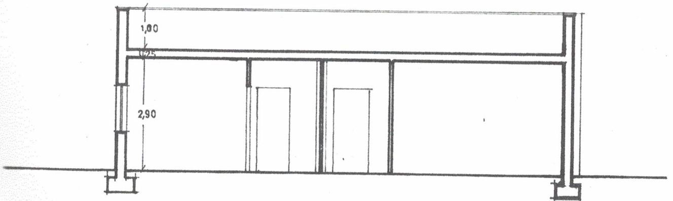
Sezione A-B
