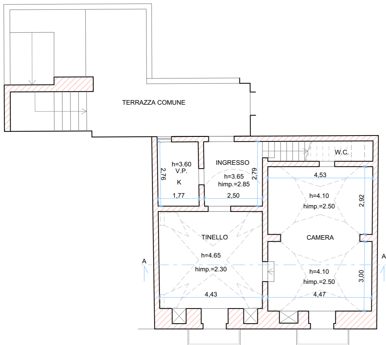
PIANTA PIANO PRIMO R. 1:100 (Stato dei Luoghi)
