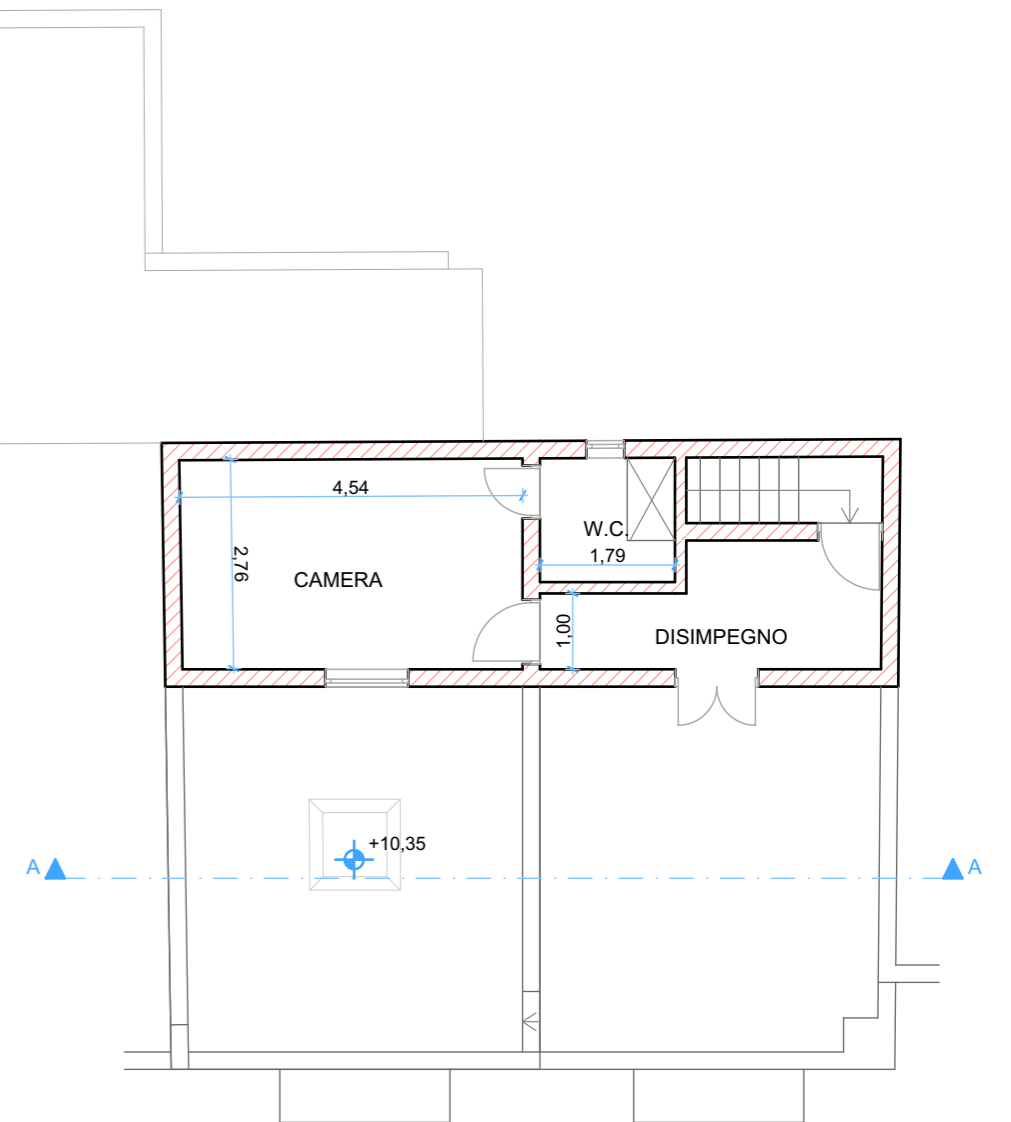
PIANTA PIANO ATTICO R. 1:100 (Di Progetto)
