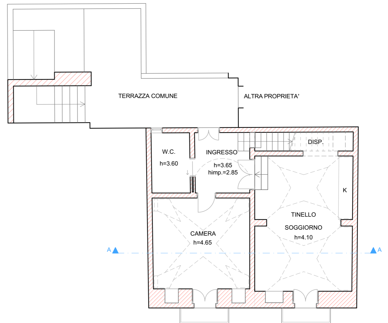
PIANTA PIANO PRIMO R. 1:100 (Di Progetto)
