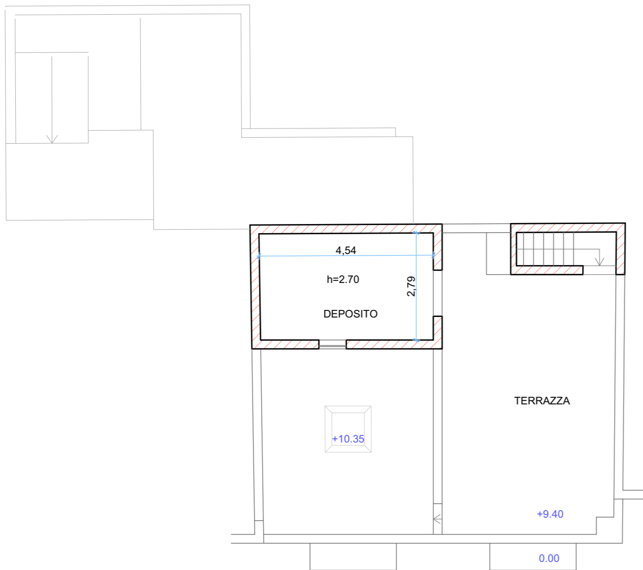
PIANTA PIANO ATTICO R. 1:100 (Stato dei Luoghi)
